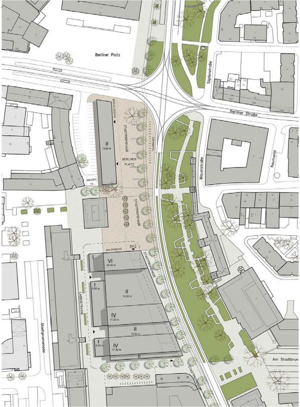
Städtebaulicher Entwurf
