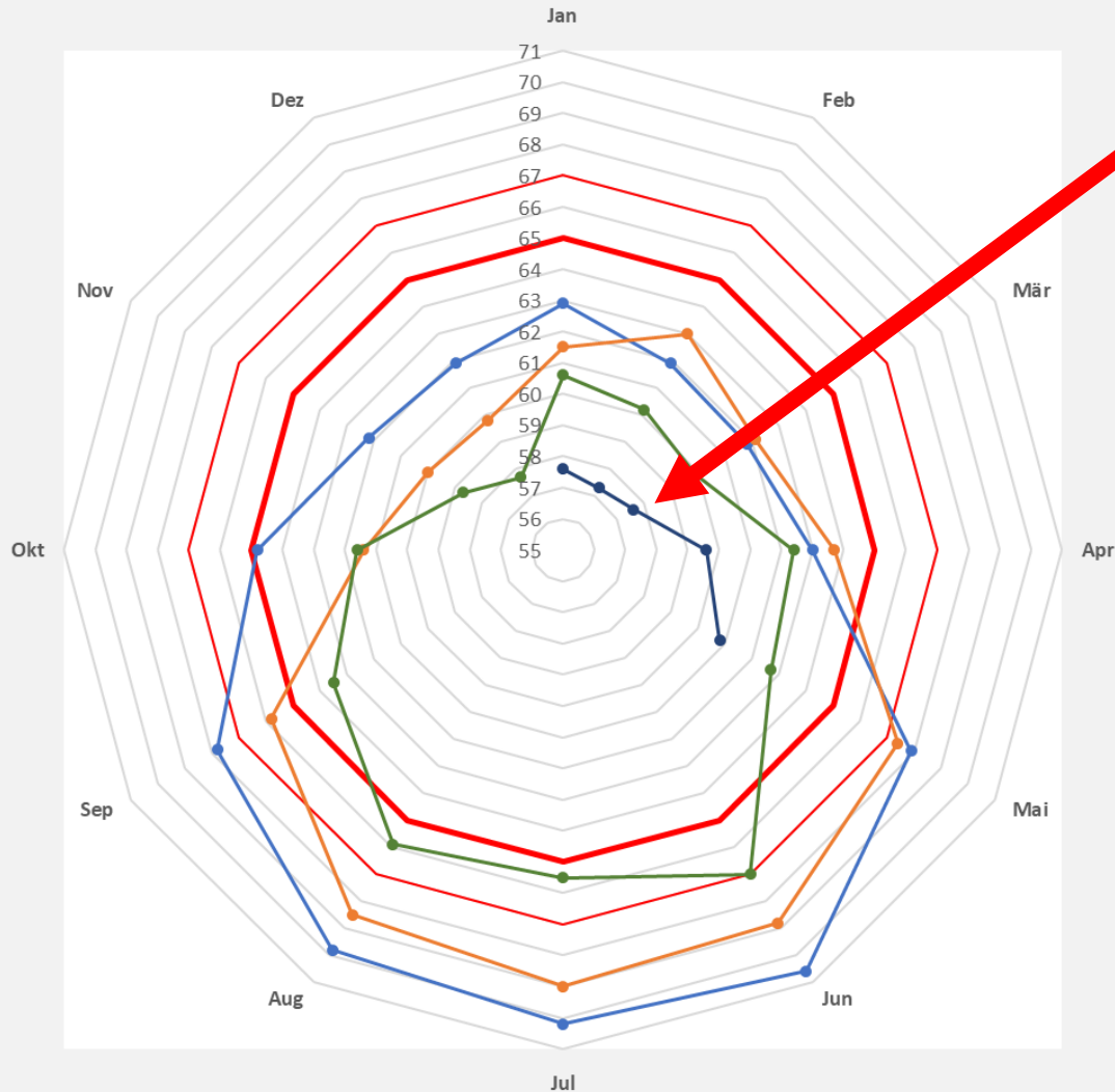
Entwicklung der mittleren Primärücklauftemperatur seit 2017 (TRL in °C)
